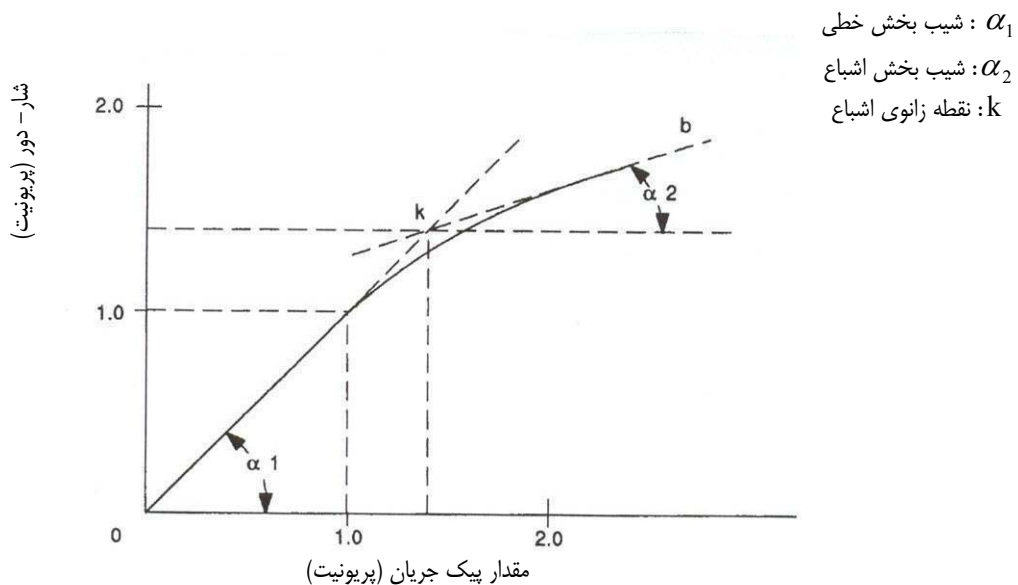
شکل ۱-۲: مشخصه غیرخطی مغناطیسی هسته
