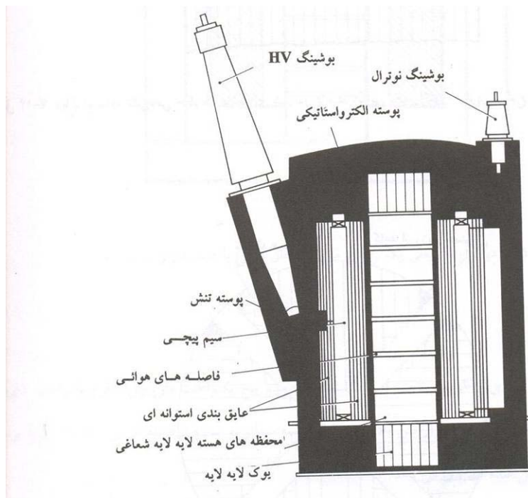
شکل ۱-۱: ساختمان یک راکتور موازی تکفاز
