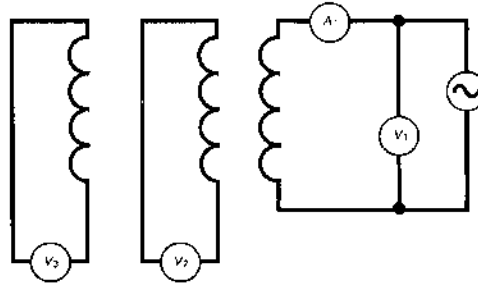
شکل ۱-۳: مدار آزمون اندازه‌گیری راکتانس متقابل
