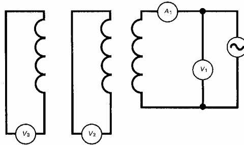
شکل ۳-۱: مدارآزمون اندازه‌گیری راکتانس متقابل
